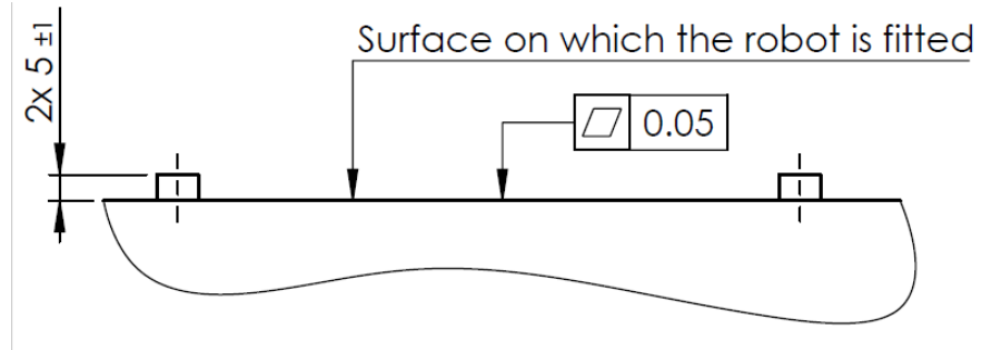
1.2: Robot tabanı için montaj plakası
